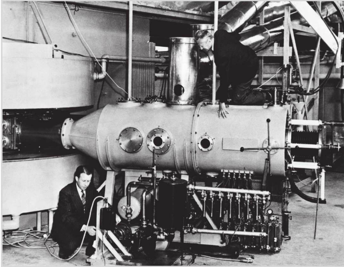
▲ 才华横溢的美国物理学家欧内斯特·劳伦斯(左下)发明了回旋加速器，用来为质子提供能量。回旋加速器将质子速度翻倍，就可作为治疗他母亲癌症的辐射枪。
